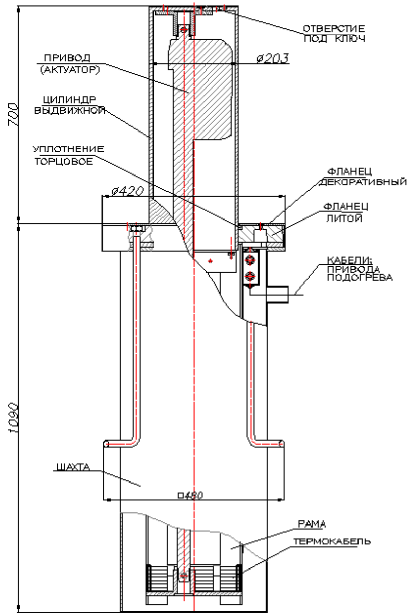
Рисунок 1. Устройство заградительного столба
