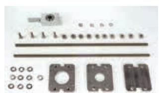
Positive Stop - механические концевые выключатели открывания/закрывания (встраиваемые в мод. 400)
