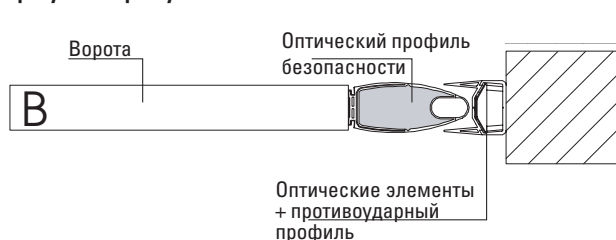
Рис. В - На противоударный профиль безопасности Требуемые артикулы 112000 + 112001 + 112002
