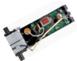
Плата управления E 550 (встроена в привод)
