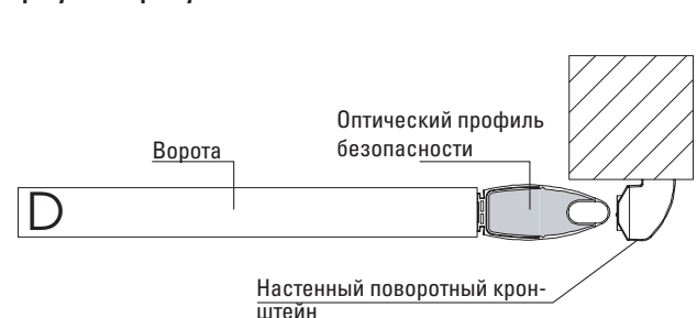
Рис. D - Монтаж с поворотным кронштейном для крепления к стене Требуемые артикулы 112000 + 112001 + 112003
